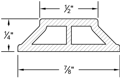
7/8" OG MUNTIN
