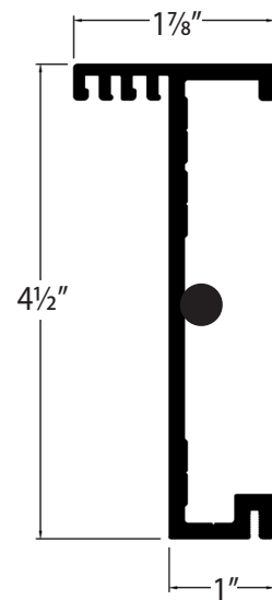
JAMB
