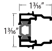
ASTRAGAL
