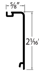
END CAP
