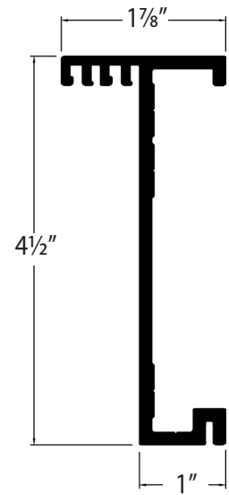
JAMB
