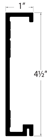
JAMB
